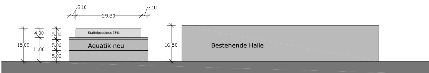
Schnitt B-B
